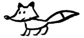
un renard
