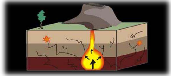
زلزال بركاني
