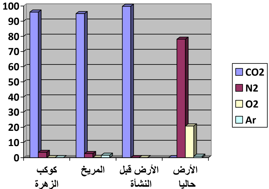
تركيب الغلاف الجوي للأرضي
