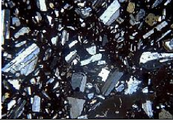
صورة لشريحة صخر الإندونيزيت تحت المجهر المستقطب
