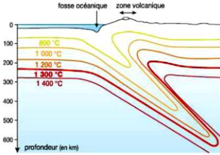
Modèle des isothermes en zone de subduction
