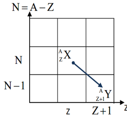
تفكك من نوع \beta^-
