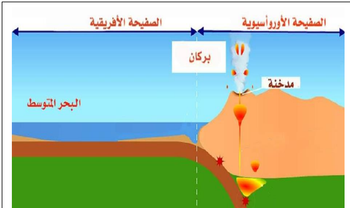
السند 2: الحدود بين الصفيحتين الإفريقية والأورواسيوية
